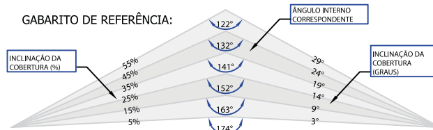
Medidas nominais
