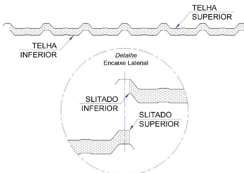
Fig.01 – Detalhe da colagem do EPS na telha.
